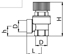
Valvola di sicurezza attacco femmina Safety valve, female connection Válvula de seguridad, empalme hembra
