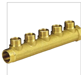
Collettore a 5 attacchi filetto maschio Manifold with 5 male outlets Colector de 5 empalmes rosca macho
